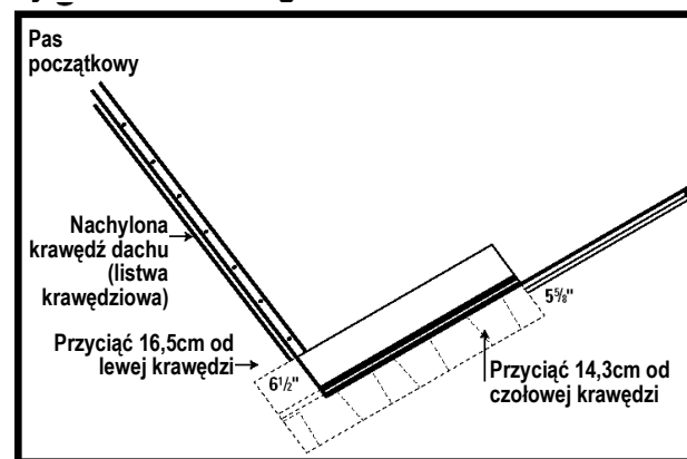
Rys. 5 Układanie gontów
